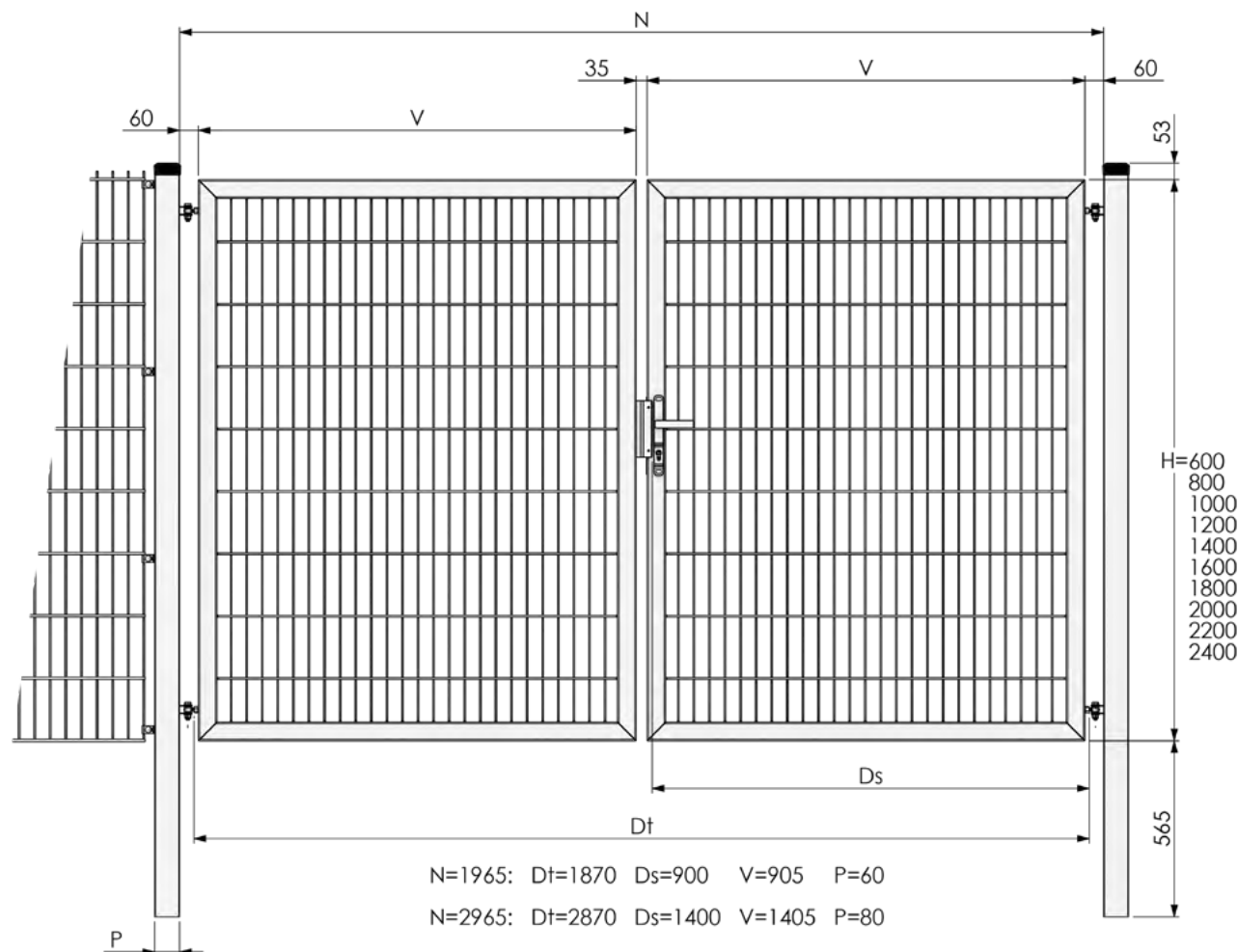
Dubbele Premium poort 2000 mm en 3000 mm
